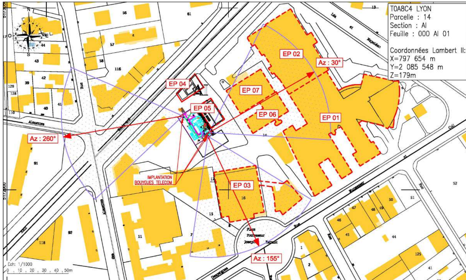
PLAN DES AZIMUTS DES ANTENNES AVEC LOCALISATION DES ESTIMATIONS DONNEES
