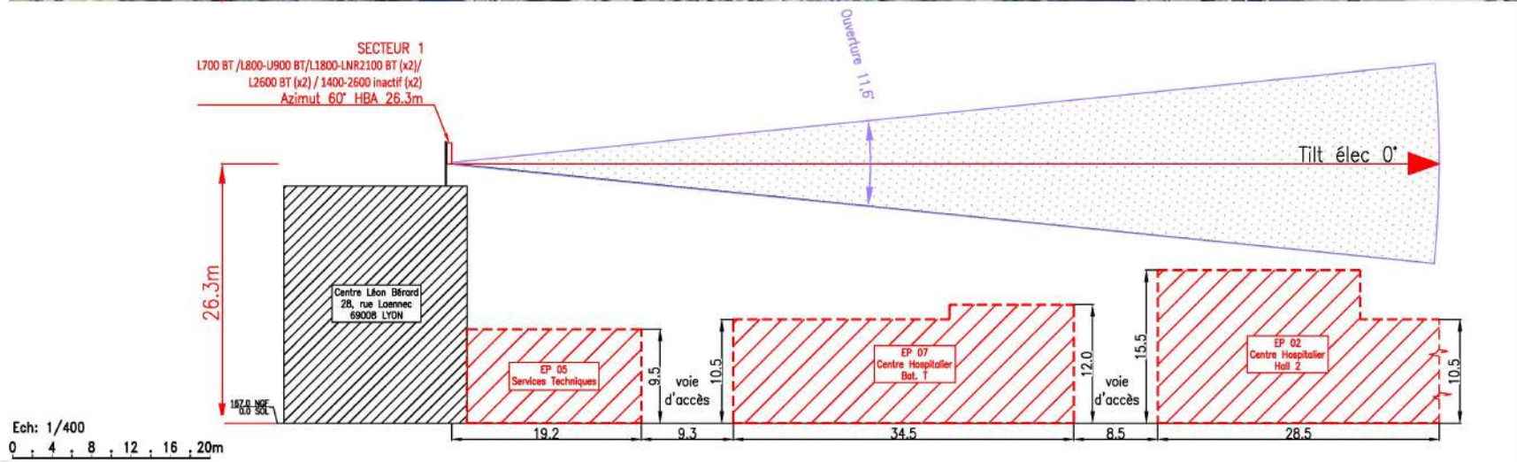
VUE EN COUPE DE L'AZIMUT 60°
