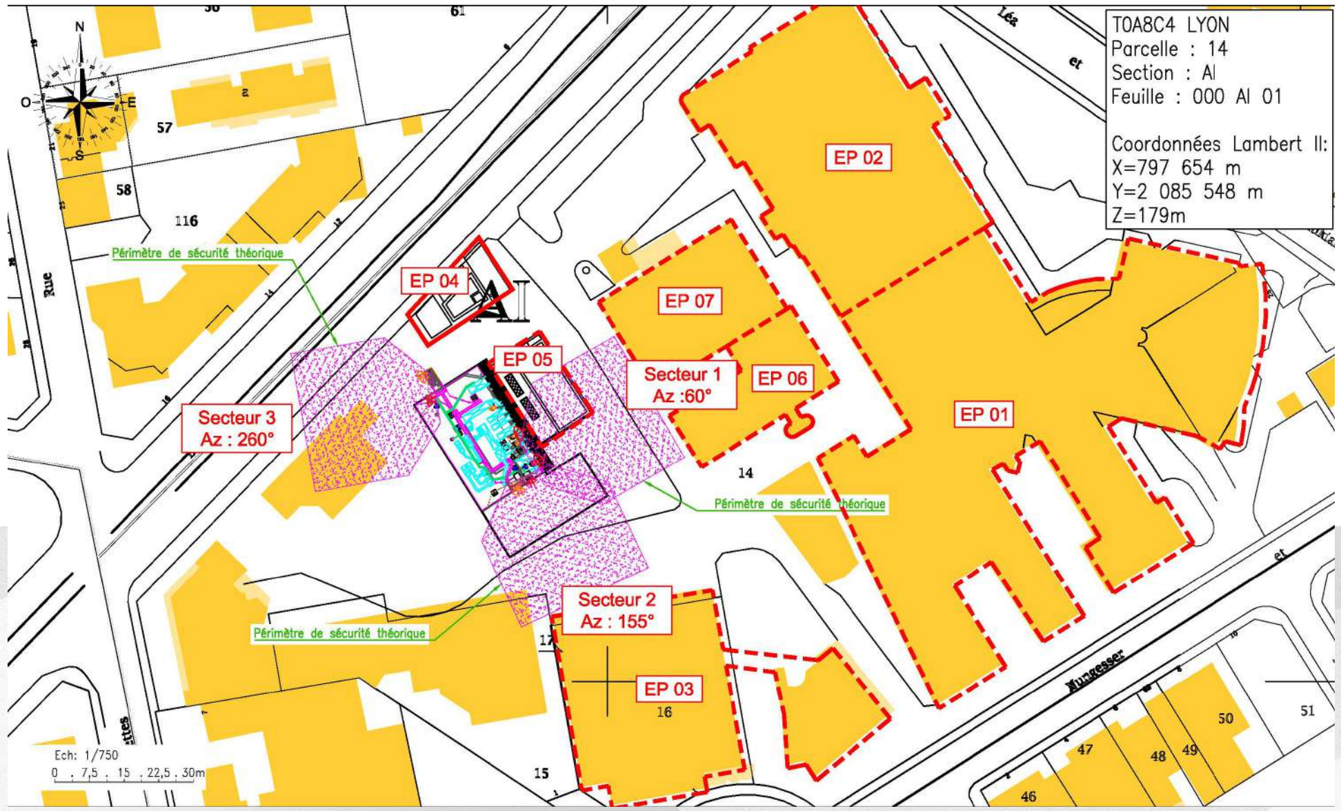
PERIMETRE DE SECURITE VUE EN PLAN
