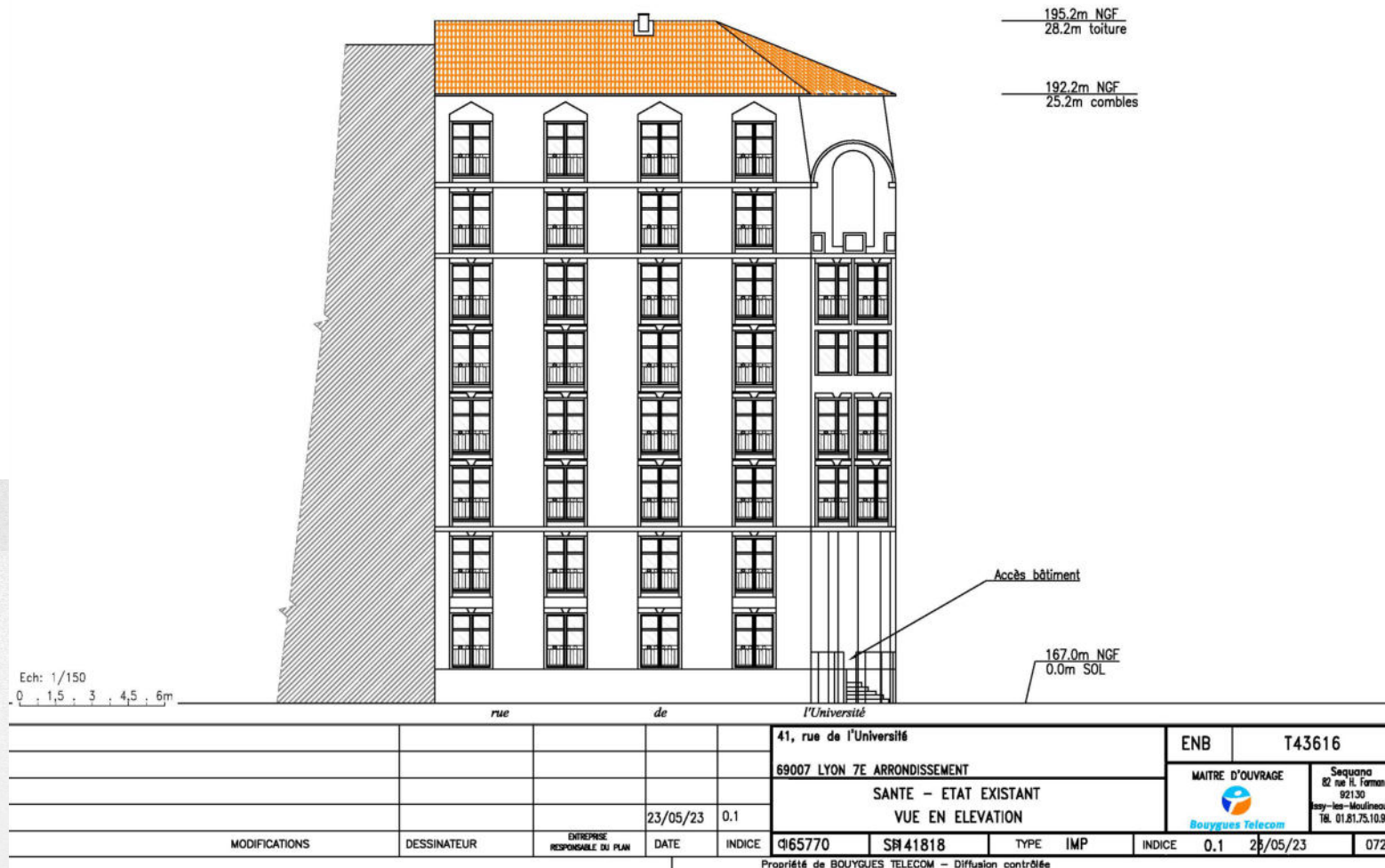
PLAN EN ELEVATION DES INSTALLATIONS EXISTANTES
