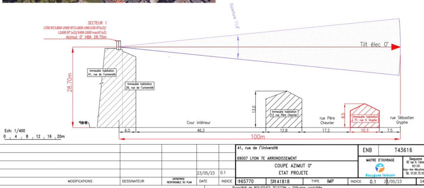
VUE EN COUPE DE L'AZIMUT 0°
