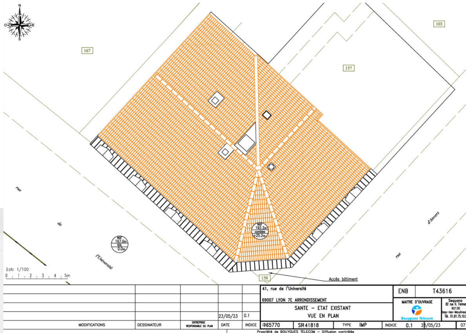
PLAN DES INSTALLATIONS EXISTANTES
