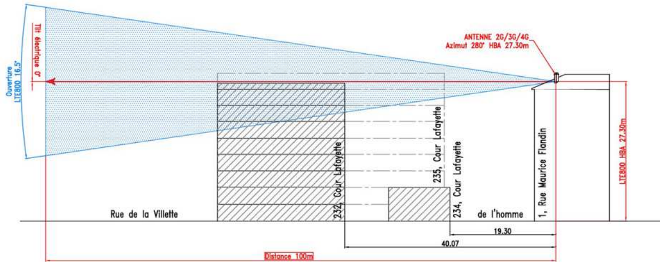
VUE EN COUPE DE L'AZIMUT 280°
