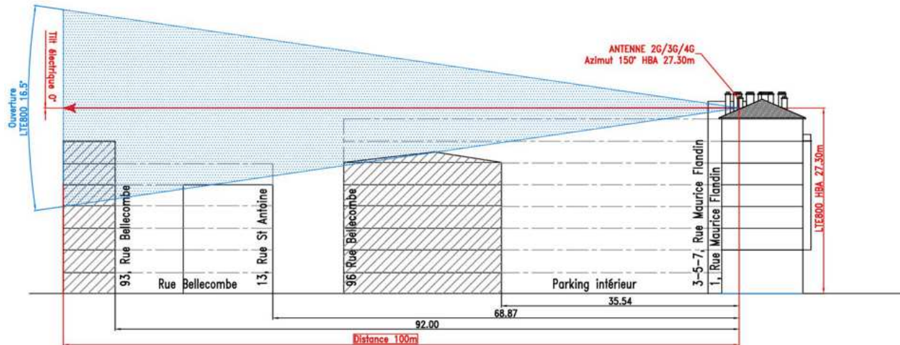
VUE EN COUPE DE L'AZIMUT 150°
