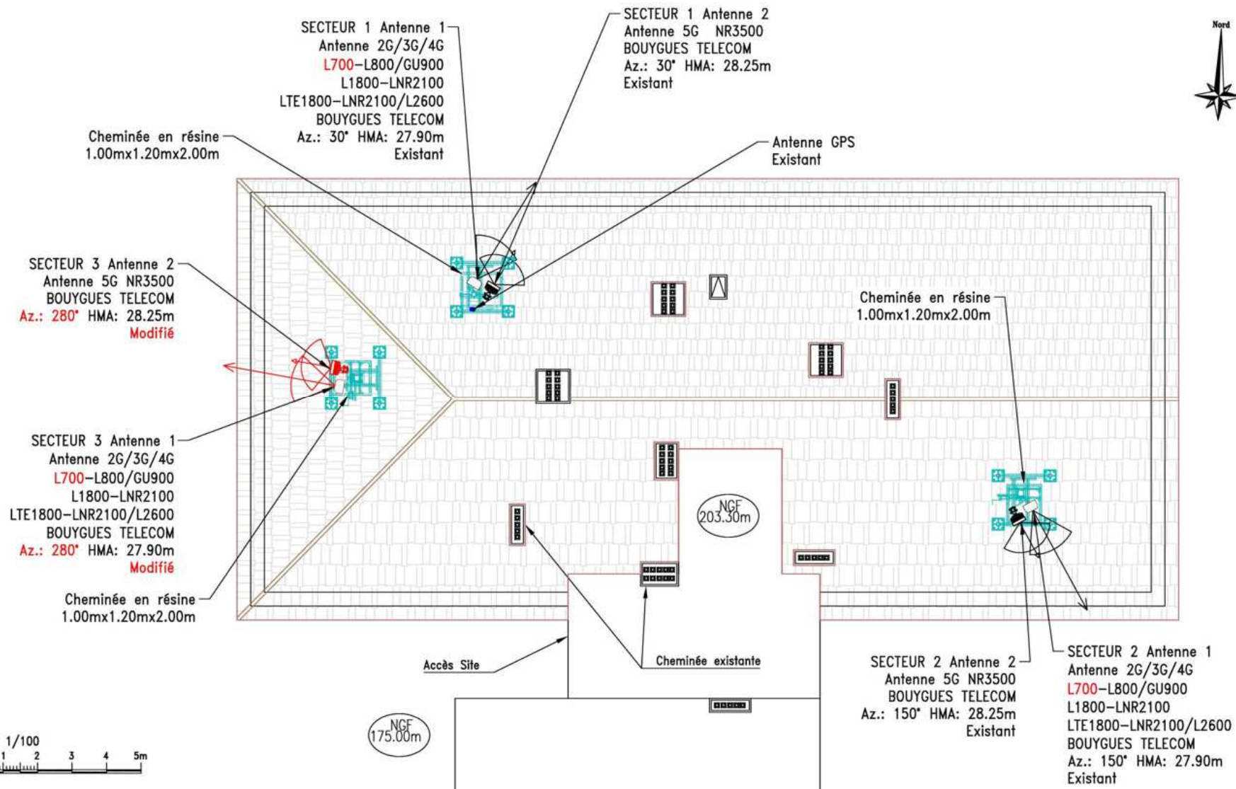
PLAN DE L'INSTALLATION BOUYGUES TELECOM
