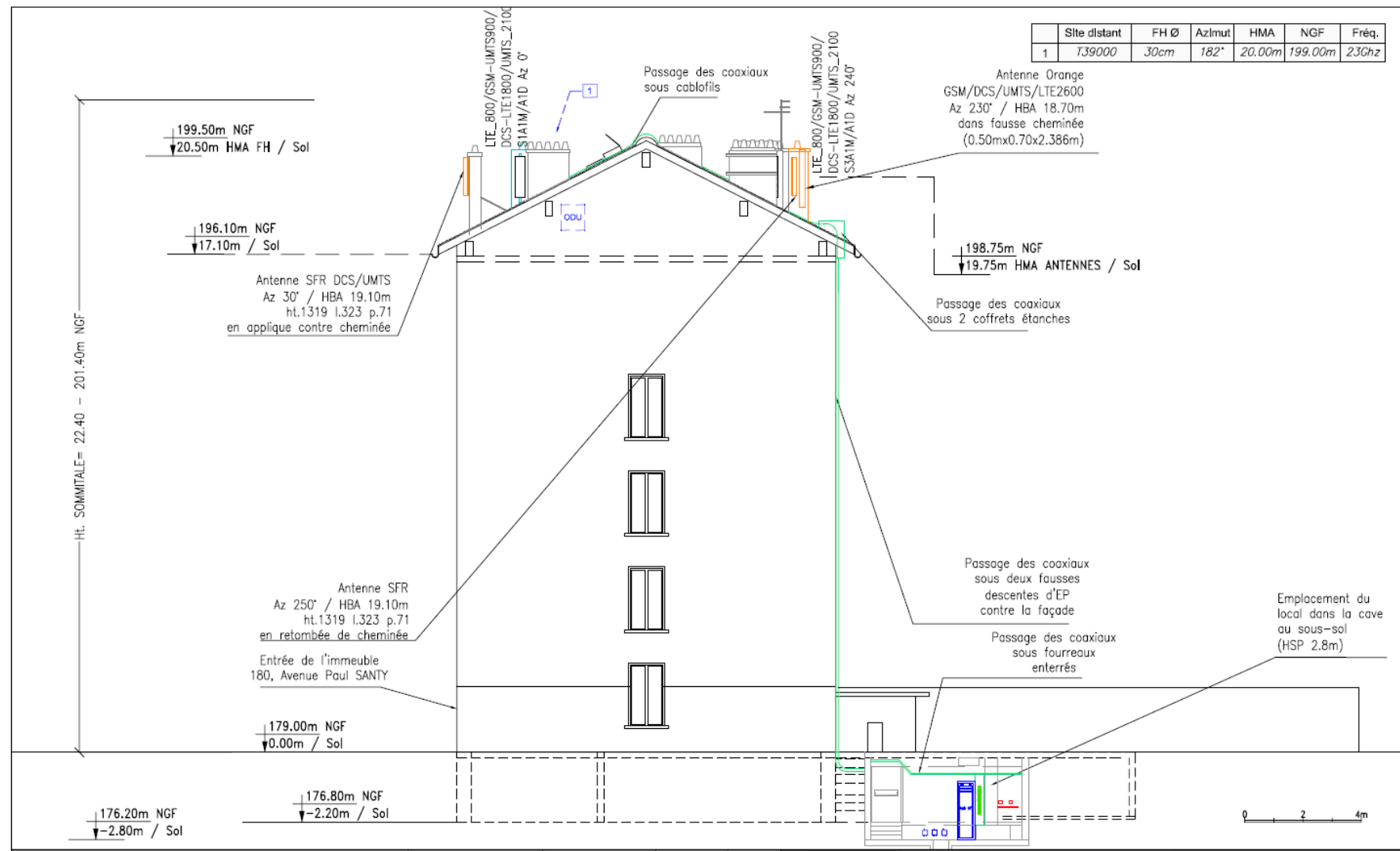
PLAN EN ELEVATION DES INSTALLATIONS EXISTANTES
