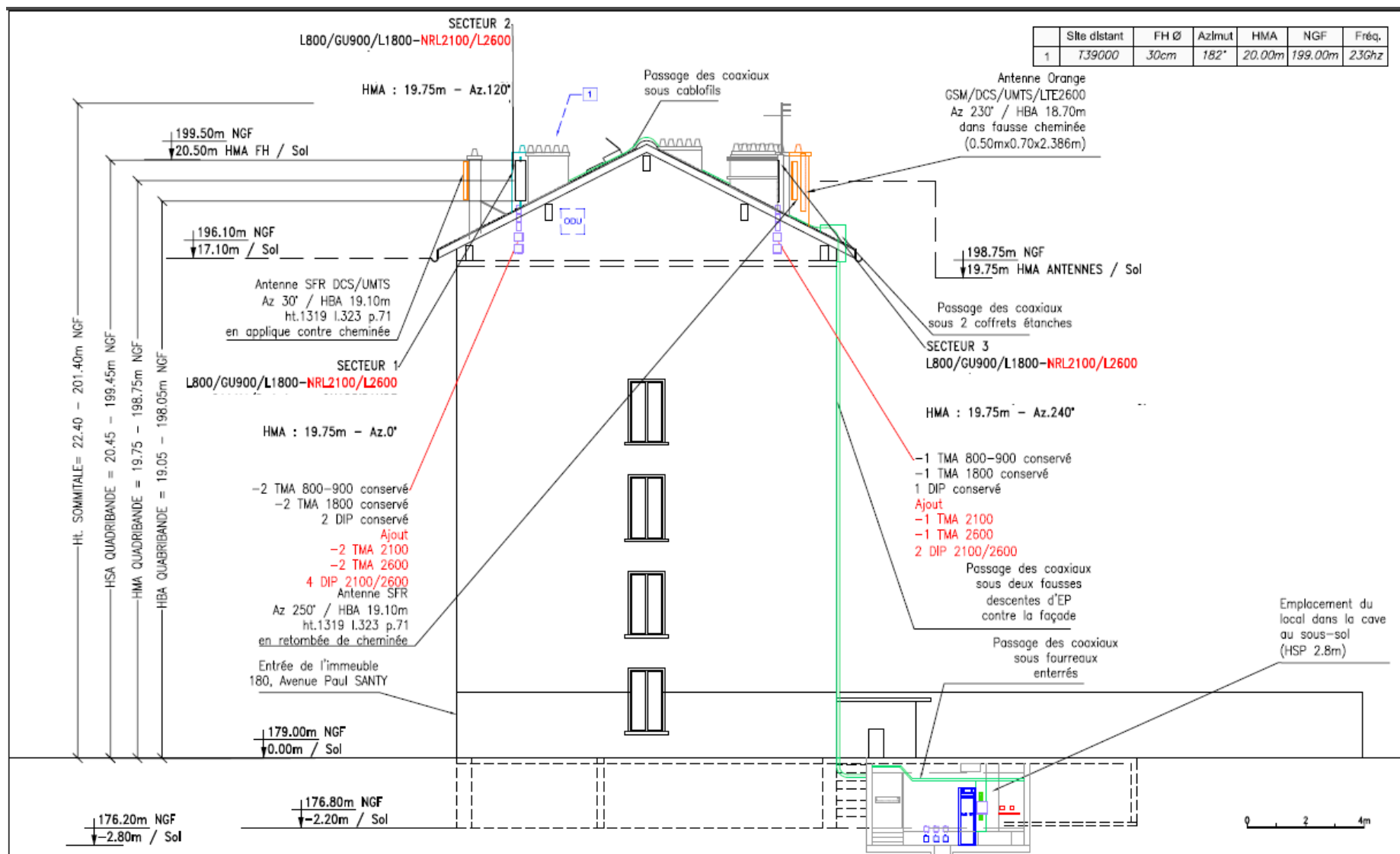
PLAN EN ELEVATION DE L'INSTALLATION BOUYGUES TELECOM
