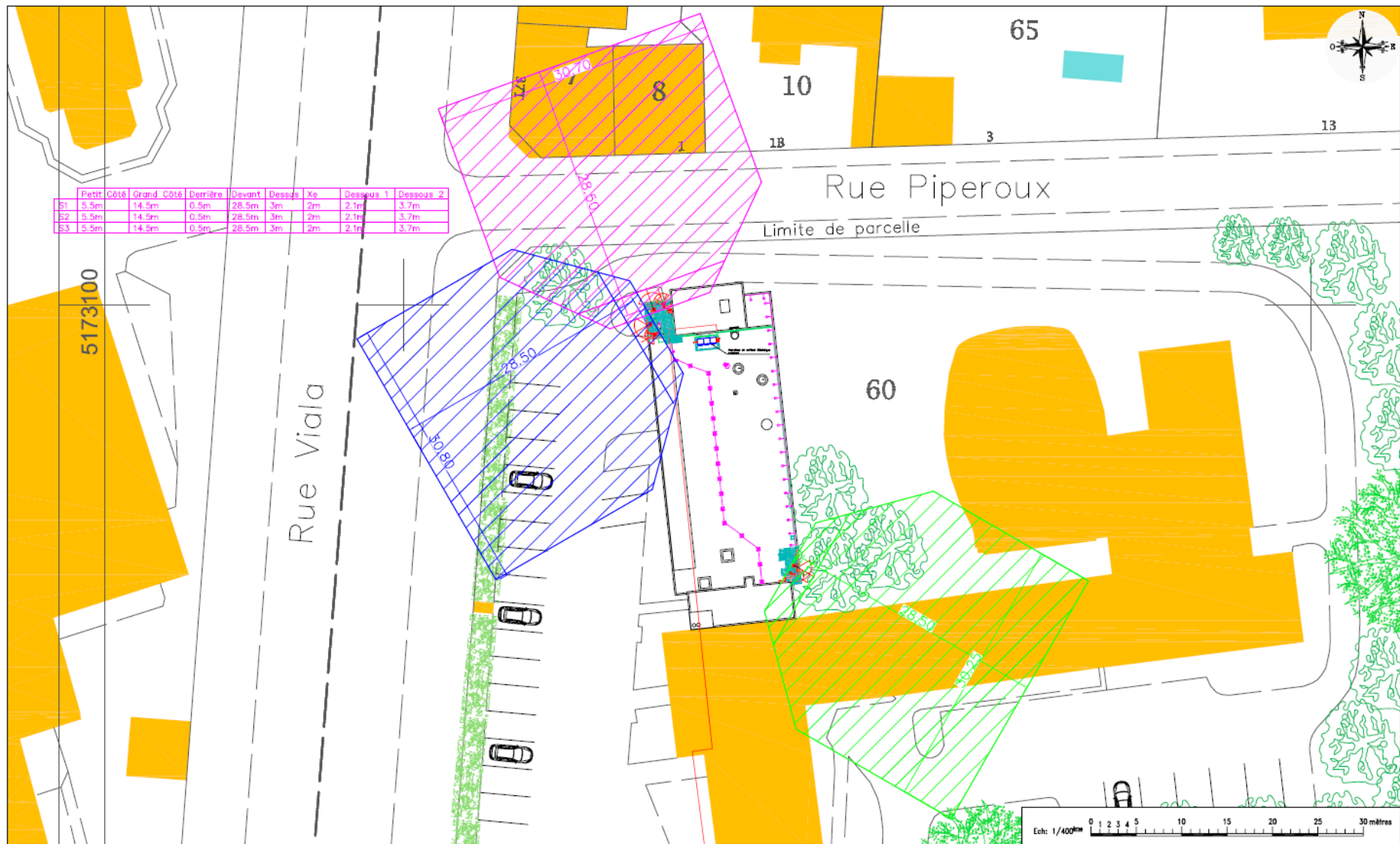
PERIMETRE DE SECURITE AUTOUR DE L'ANTENNE
