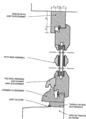
Coupe
