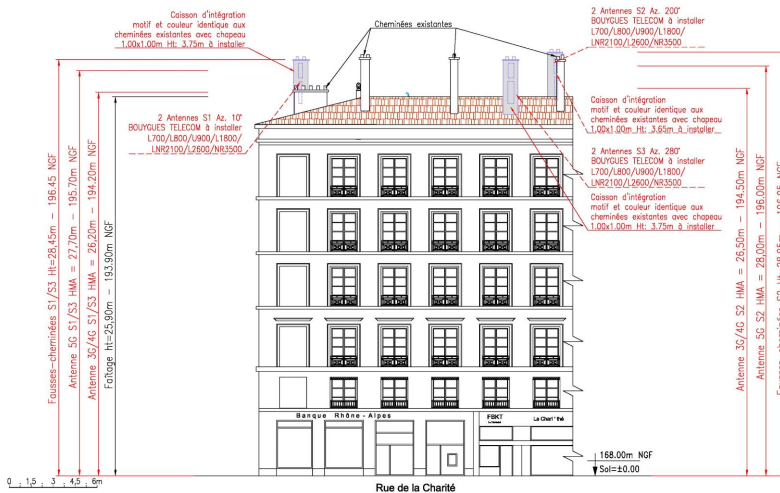
PLAN EN ELEVATION DE L'INSTALLATION BOUYGUES TELECOM
