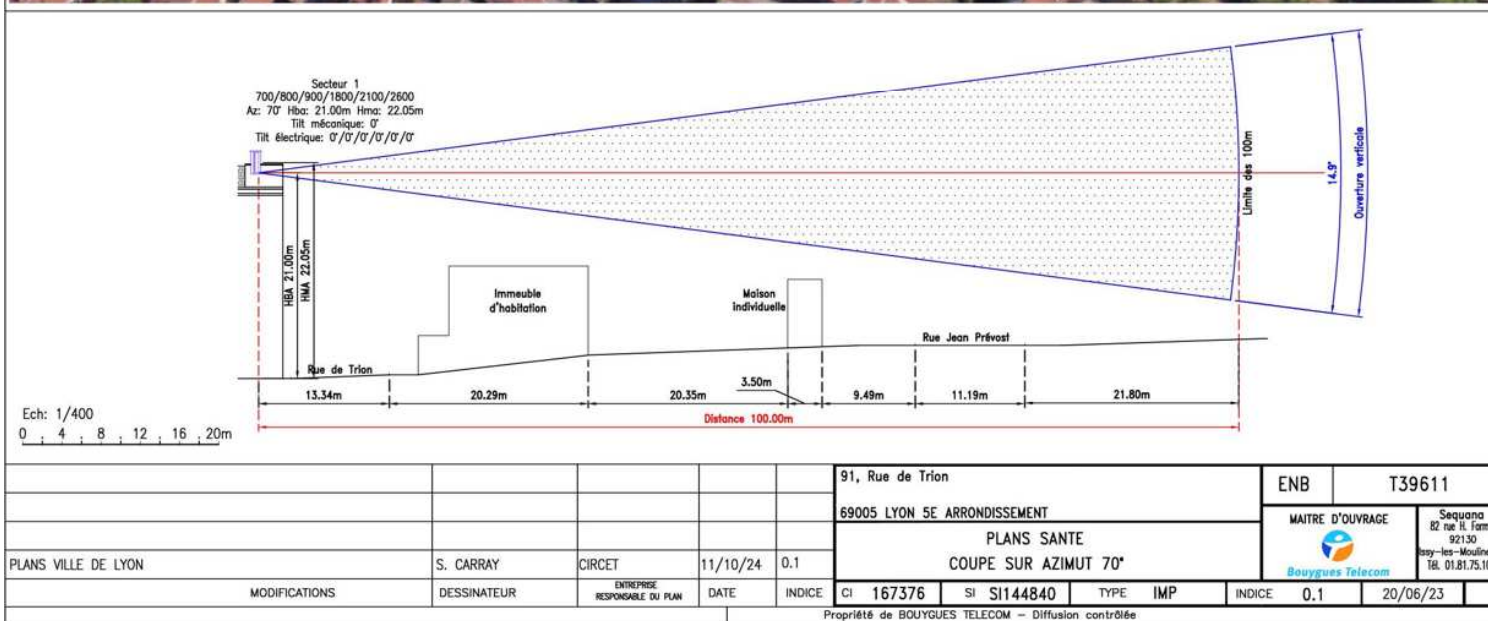
VUE EN COUPE DU SECTEUR 1 AZIMUT 70°
