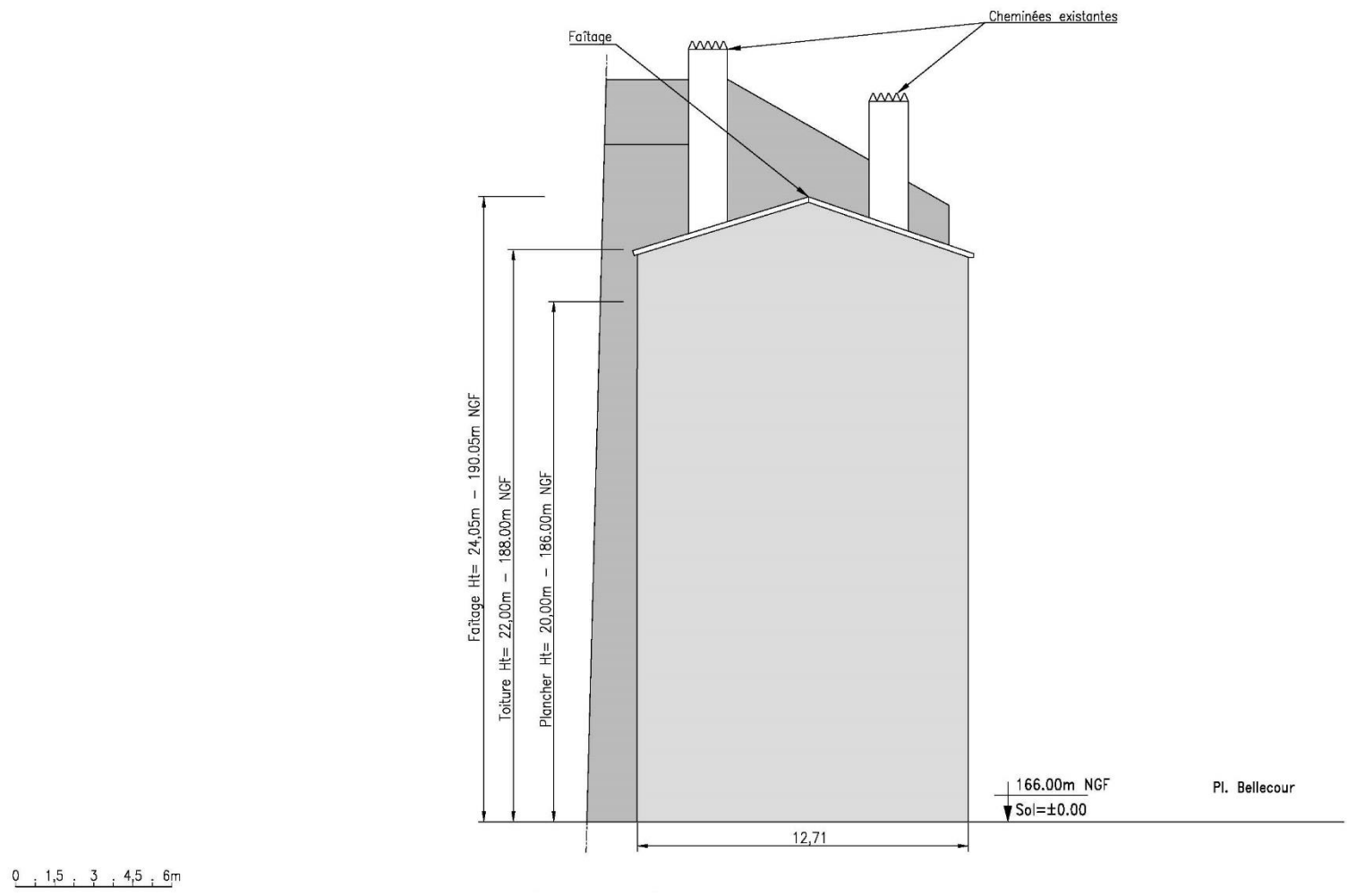
PLAN EN ELEVATION DES INSTALLATIONS EXISTANTES
