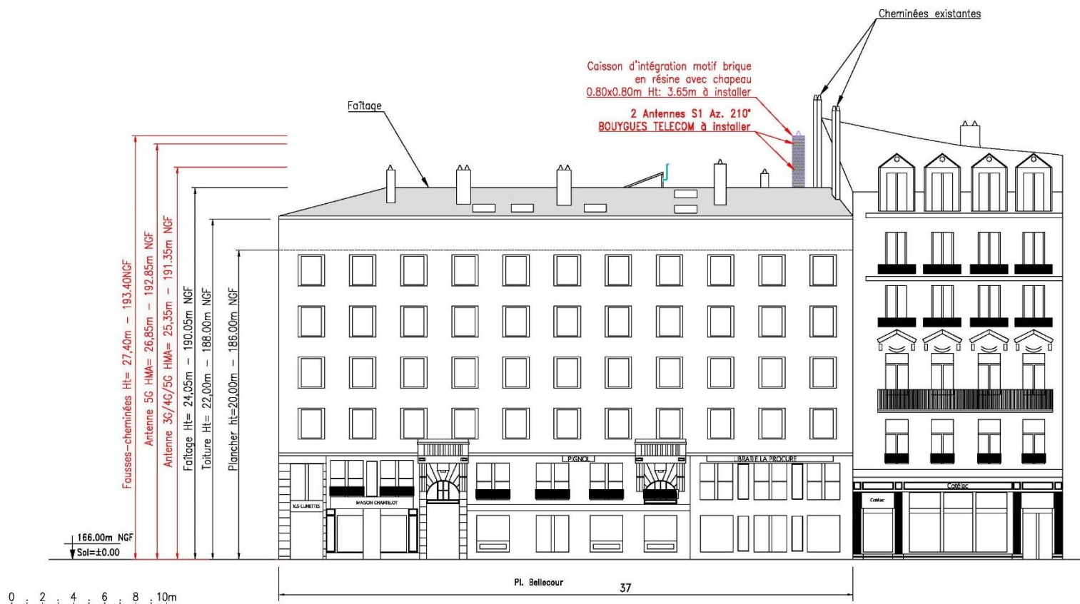
PLAN EN ELEVATION DE L'INSTALLATION BOUYGUES TELECOM
