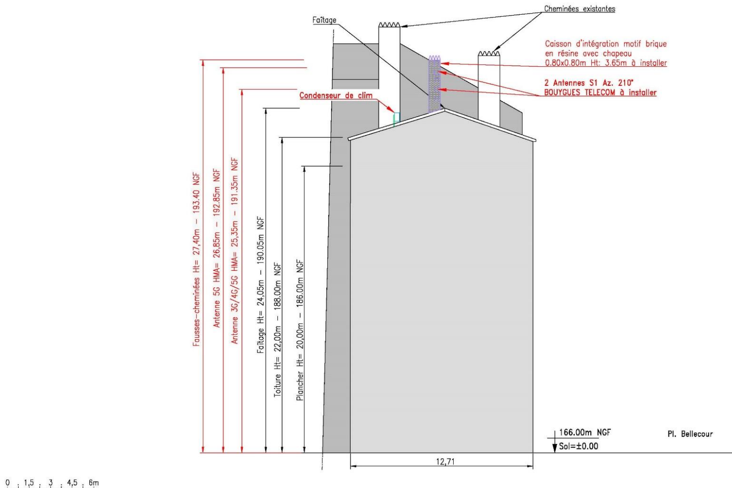
PLAN EN ELEVATION DE L'INSTALLATION BOUYGUES TELECOM
