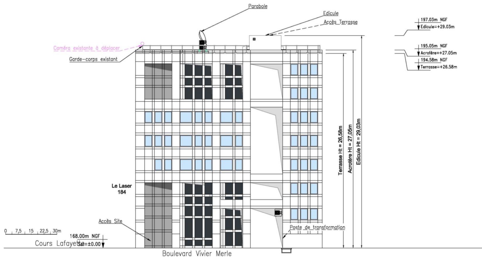
PLAN DE L'INSTALLATION BOUYGUES TELECOM
