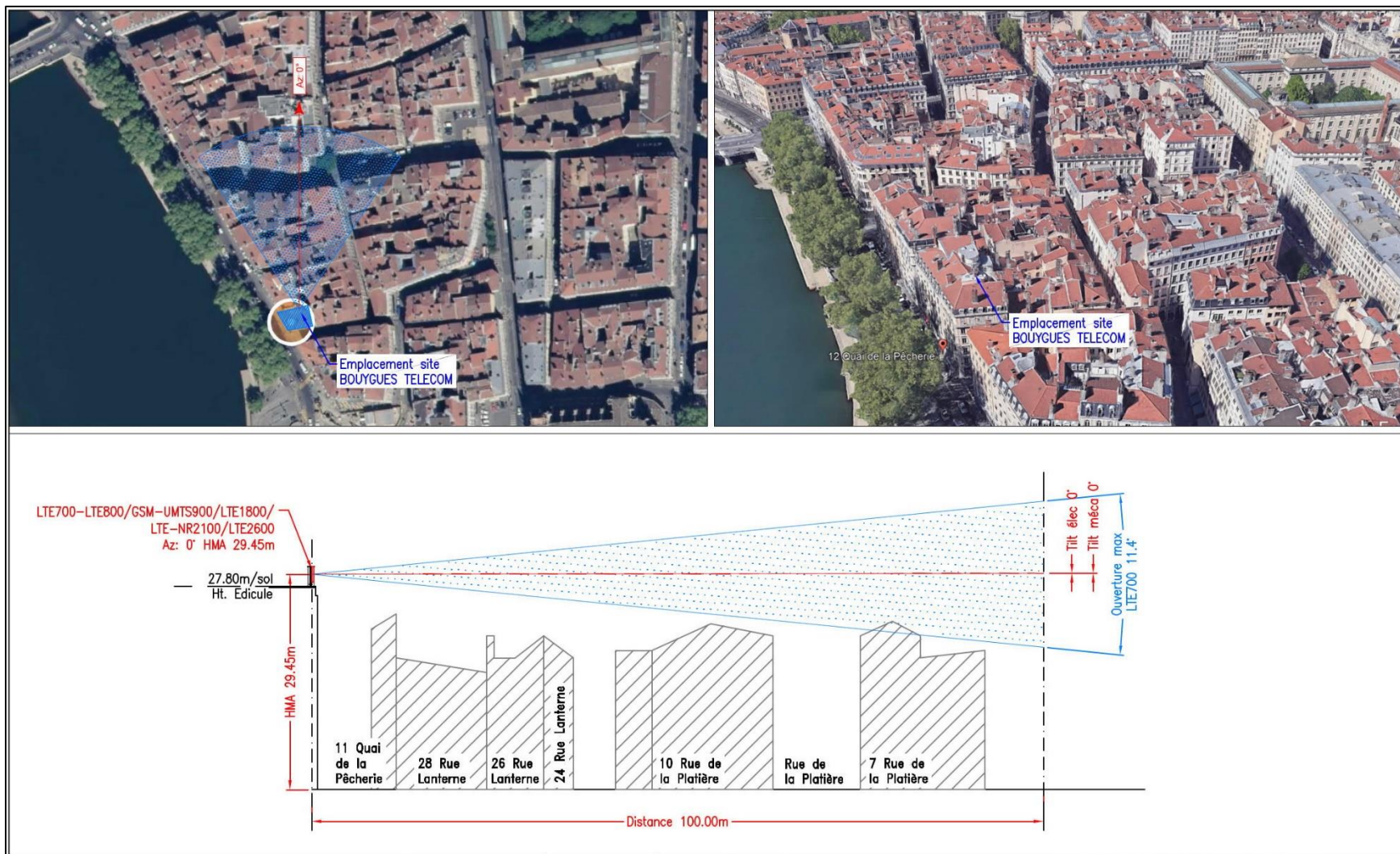
VUE EN COUPE DE L'AZIMUT 0°
