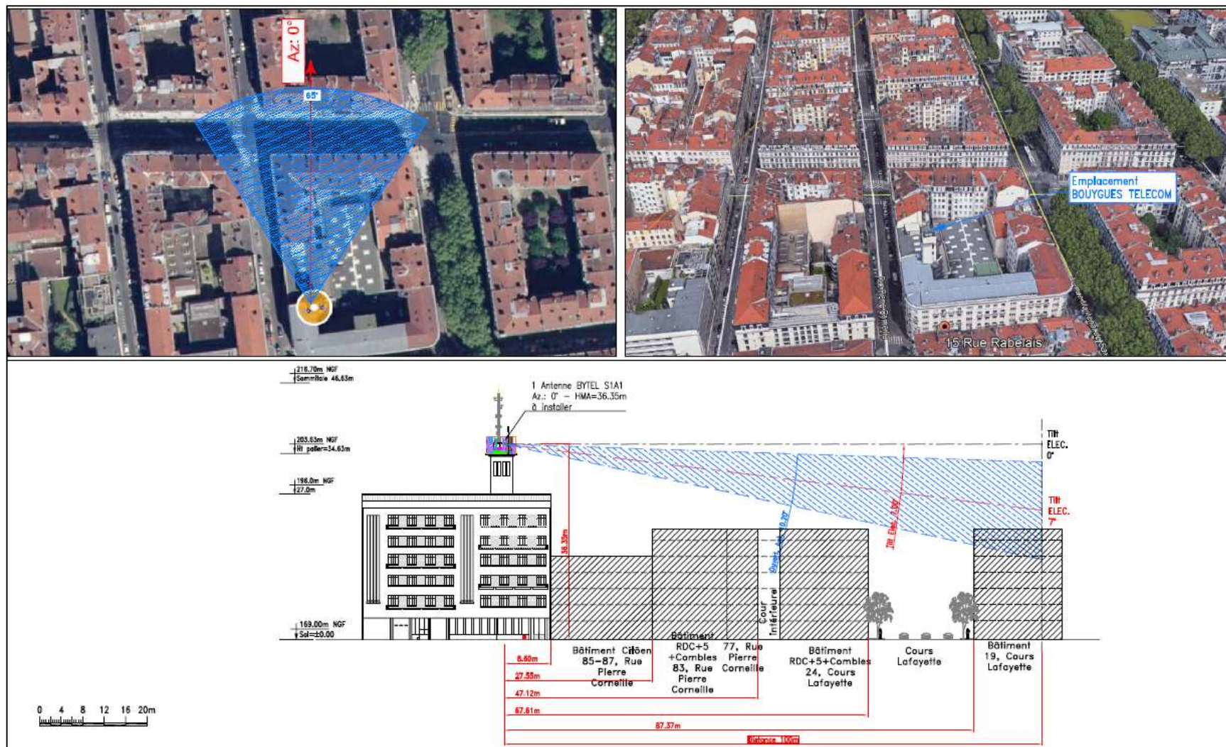
COUPE SUR L'AZIMUT 0^\circ
