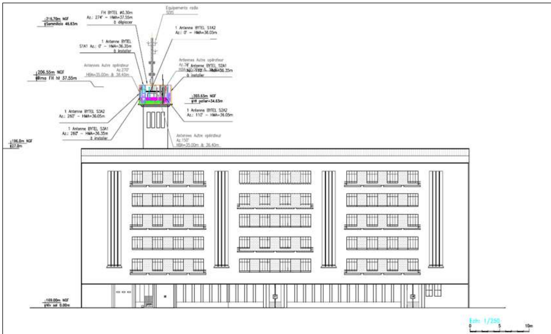
VUE EN ELEVATION ETAT PROJETE
