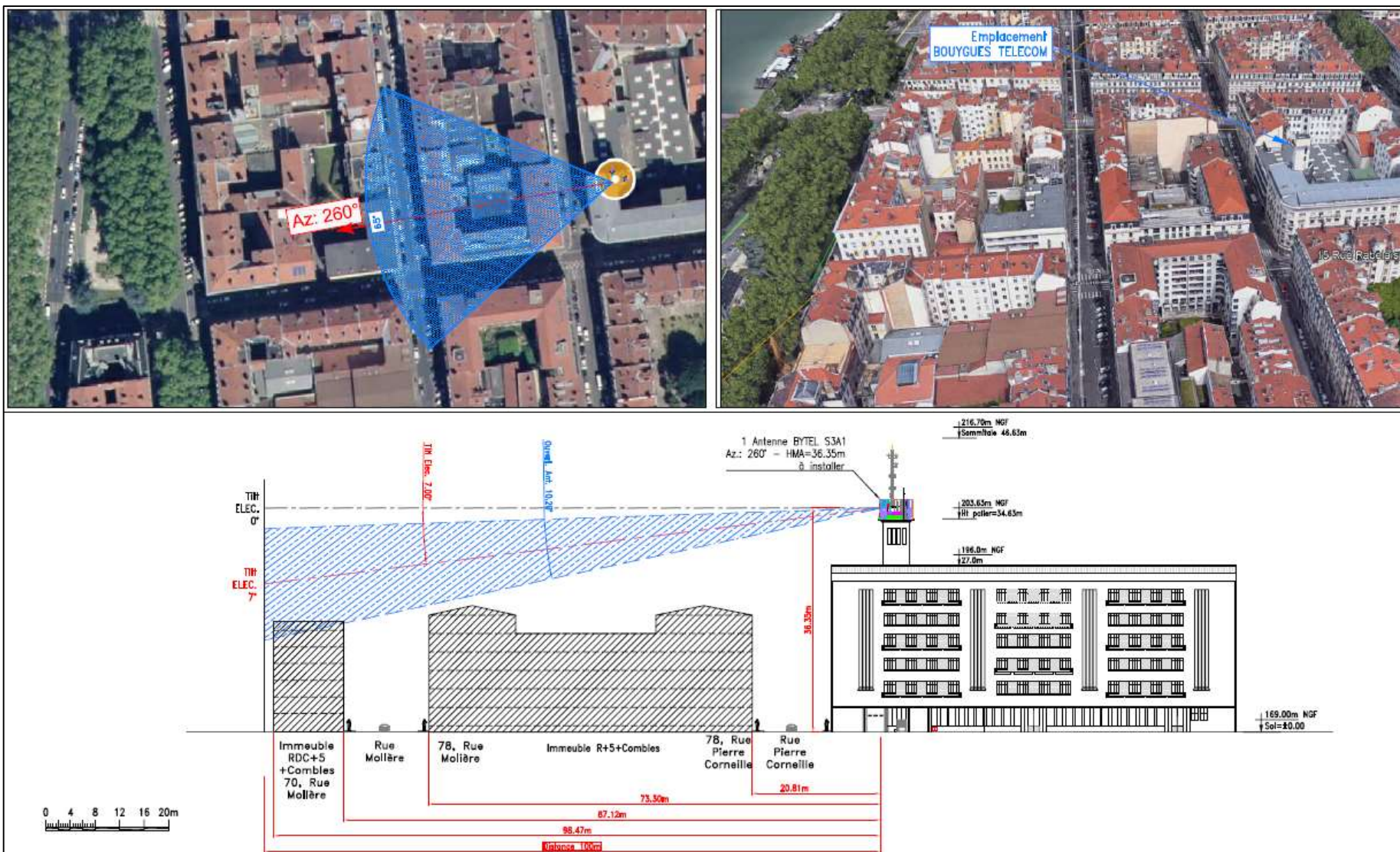
COUPE SUR L'AZIMUT 260°
