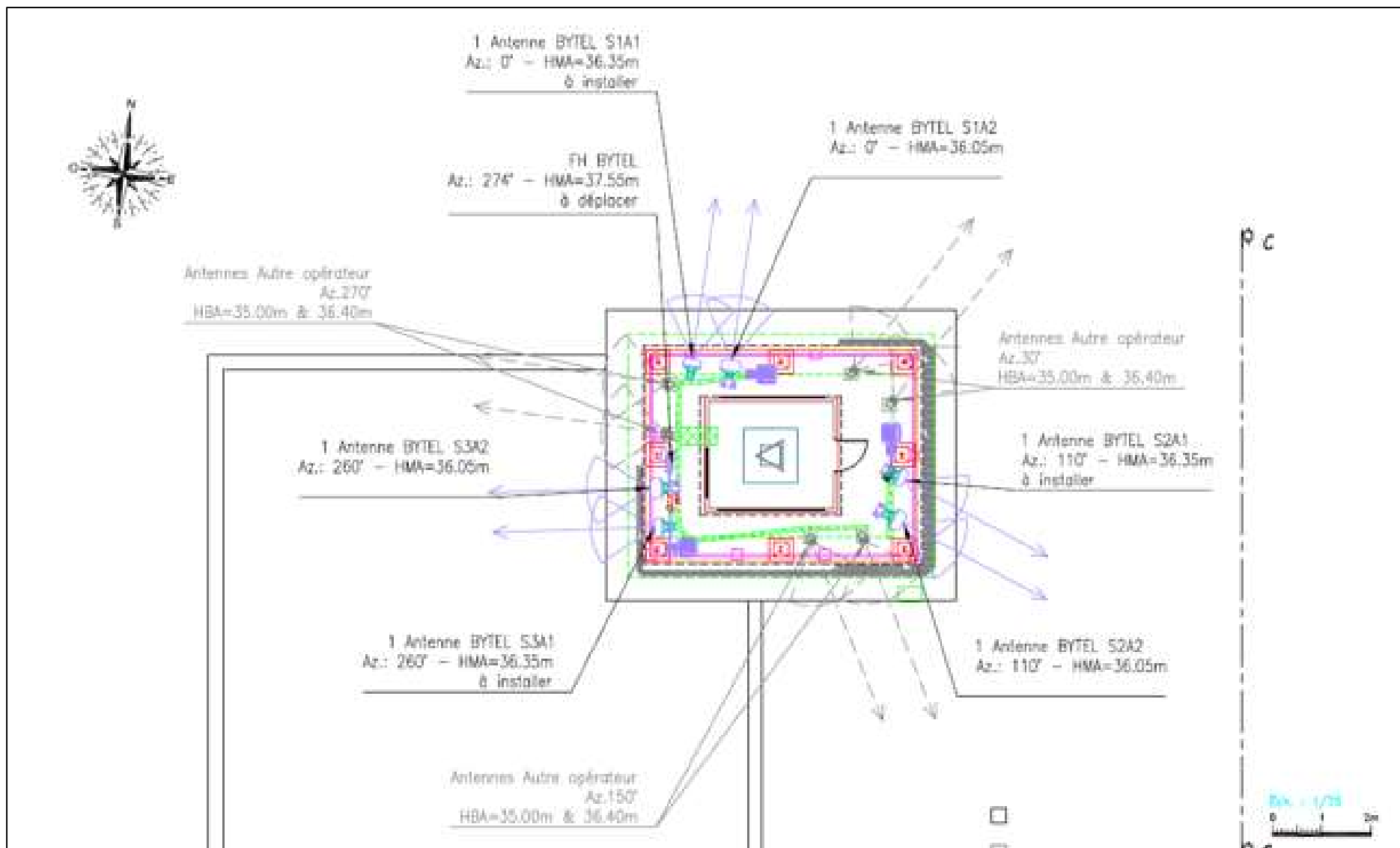
PLAN DE MASSE ETAT PROJETE
