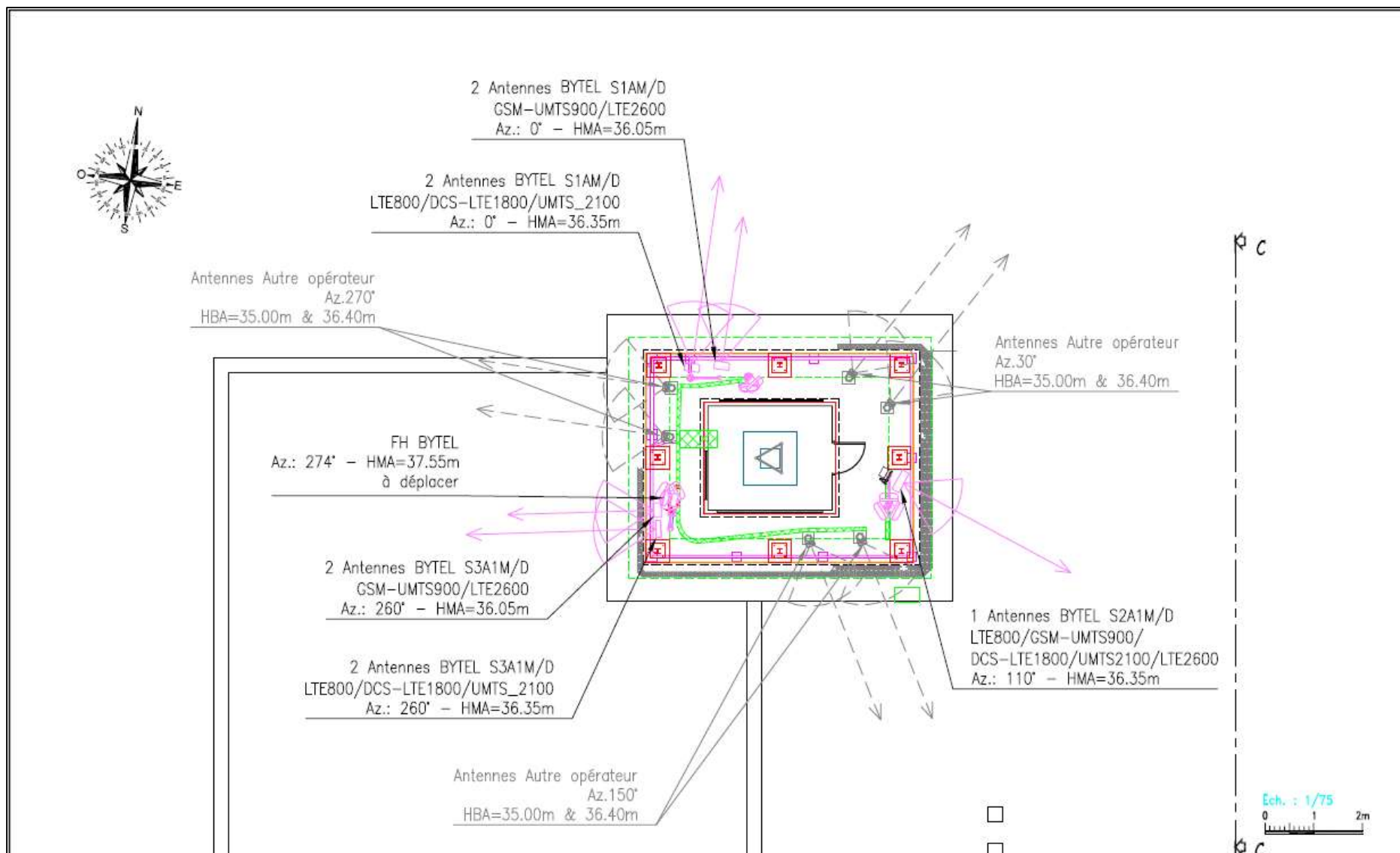
PLAN DE MASSE ETAT EXISTANT
