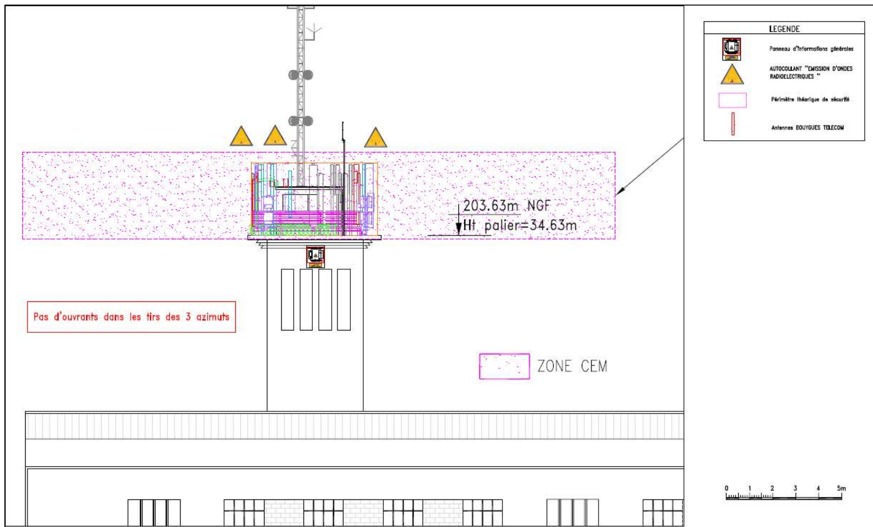
DISTANCE AUX OUVRANTS POUR CHAQUE AZIMUT
